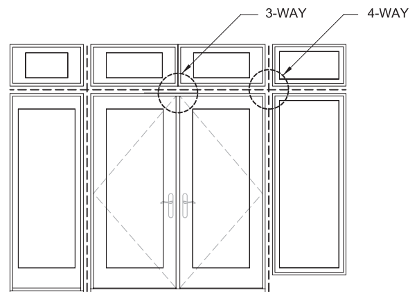
Door / Sidelight / Transom
