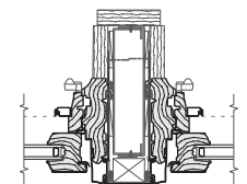
JJ - 20 ga. 1-3/8" x 6" Nested Steel Stud
