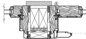
DD - (2) - 2 x 4 Wood
