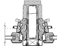
JJ - 20 ga. 1-3/8" x 6" Nested Steel Stud
