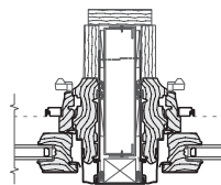
JJ - 20 ga. 1-3/8" x 6" Nested Steel Stud
