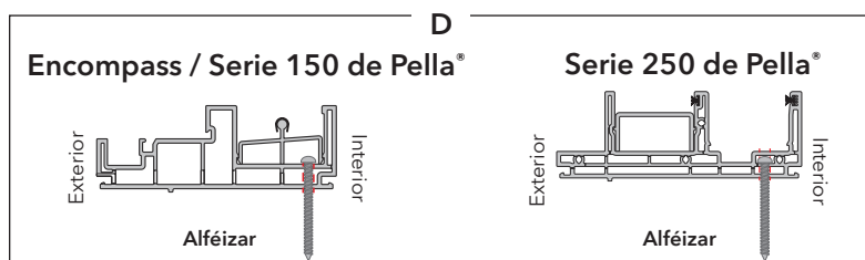
ALETA DE SUJECCIÓN DEL ALFÉIZAR RETIRADA - ANCLAJE CON TORNILLO PARA MARCO
