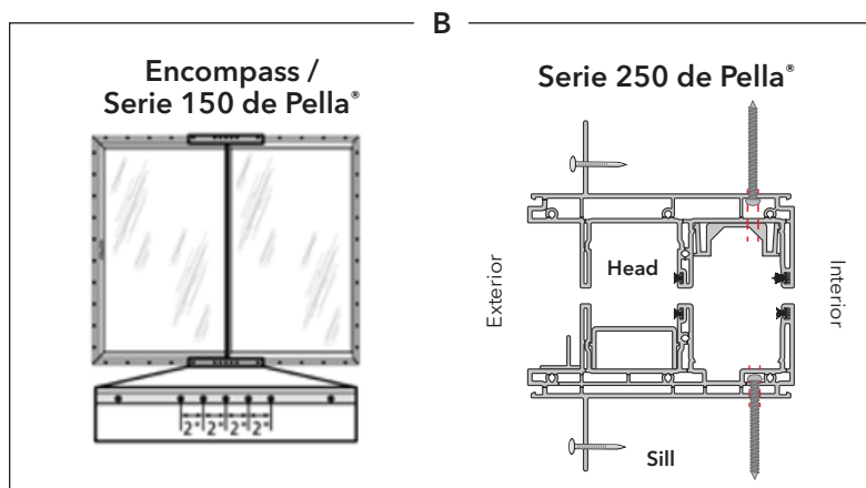
ALETA DE SUJECCIÓN DEL ALFÉIZAR RETIRADA - ANCLAJE CON TORNILLO PARA MARCO
