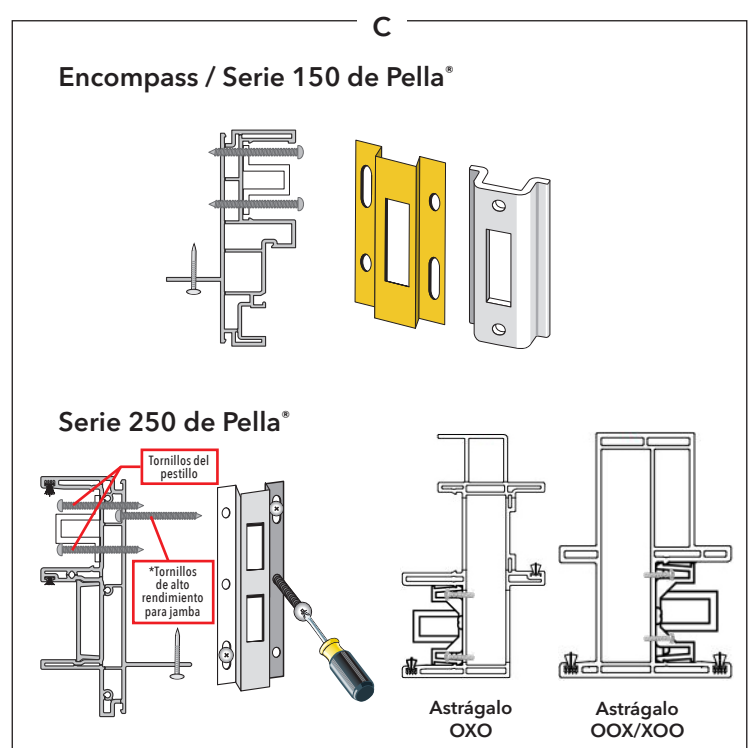
ALETA DE SUJECCIÓN DEL ALFÉIZAR RETIRADA - ANCLAJE CON TORNILLO PARA MARCO
